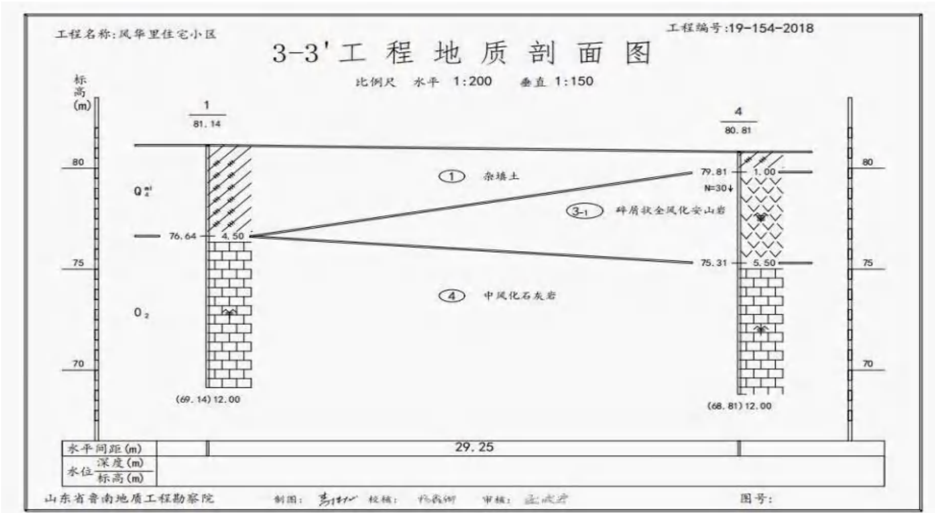
图 3.1-9 (c) 工程地质剖面图
