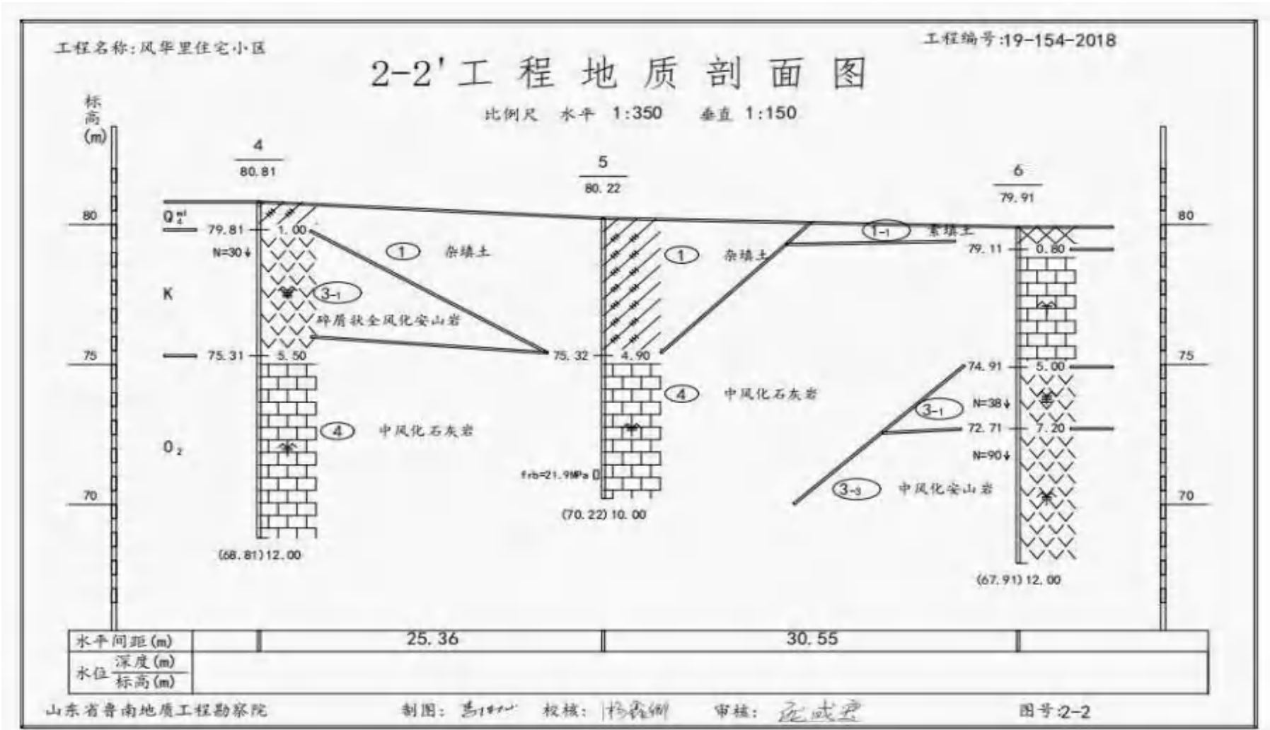
图 3.1-9 (b) 工程地质剖面图
