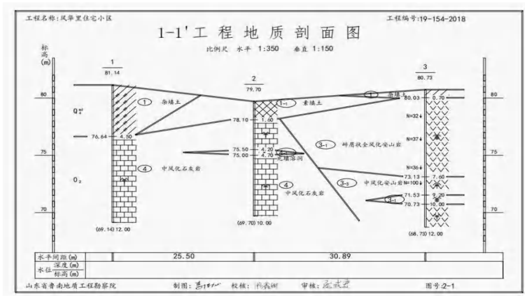
图 3.1-9 (a) 工程地质剖面图
